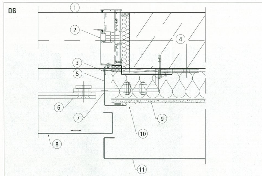
06 > Detail ostění okna, vodorovný řez
