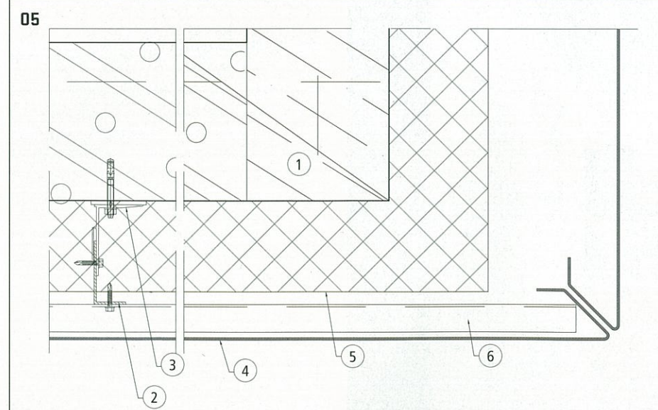
05 > Detail nároží, vodorovný řez
